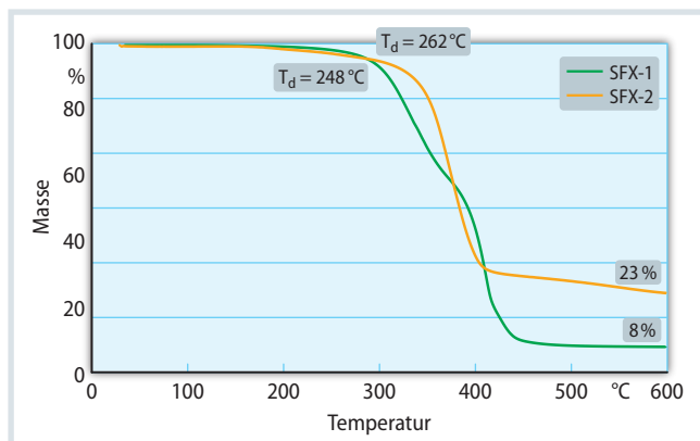
Bild 1. In der thermogravimetrischen Analyse lassen sich die verschiedenen Wirkmechanismen der Flammschutzmittel ableiten. SFX-1 ist eher in der Gasphase aktiv, SFX-2 stärker in der kondensierten Phase
