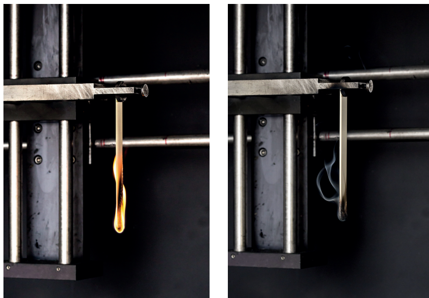
Bild 2. Prüfstab aus einem Compound mit den neu entwickelten Flammschutzmitteln während (links) und nach (rechts) der UL-94-Vertikalbrandprüfung: Die biobasierten Flammschutzmittel schneiden selbst bei geringeren zugesetzten Mengen besser ab, als verfügbare fossile Zusatzstoffe © Fraunhofer LBF
